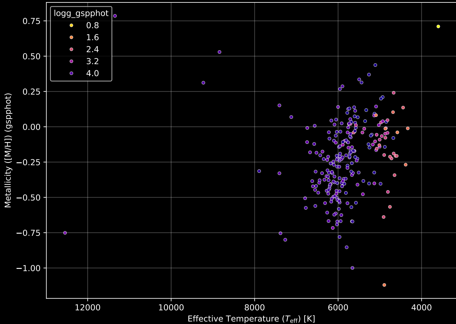
GALAH DR4 Field: [7127] Stellar Population Parameters (n= 236)
