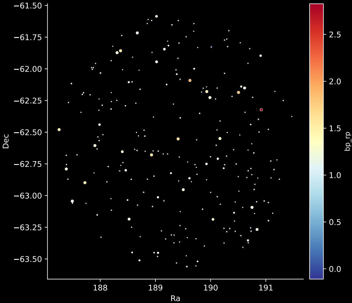
GALAH DR4 Field: [7127] Stars: 236
